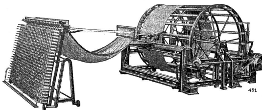
Kombinierte Seidenschner- und Aufbäummaschine, Modell mit großem Haspel
