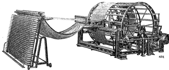
Kombinierte Seidenschere- und Aufbäummaschine, Modell mit großem Haspel
