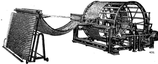
Kombinierte Seidenschner- und Aufbaumaschine, Modell mit großem Haspe
