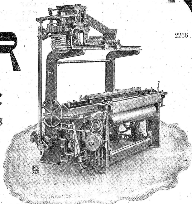
Einschifflicher Seidenwebstuhl Modell GCW.
