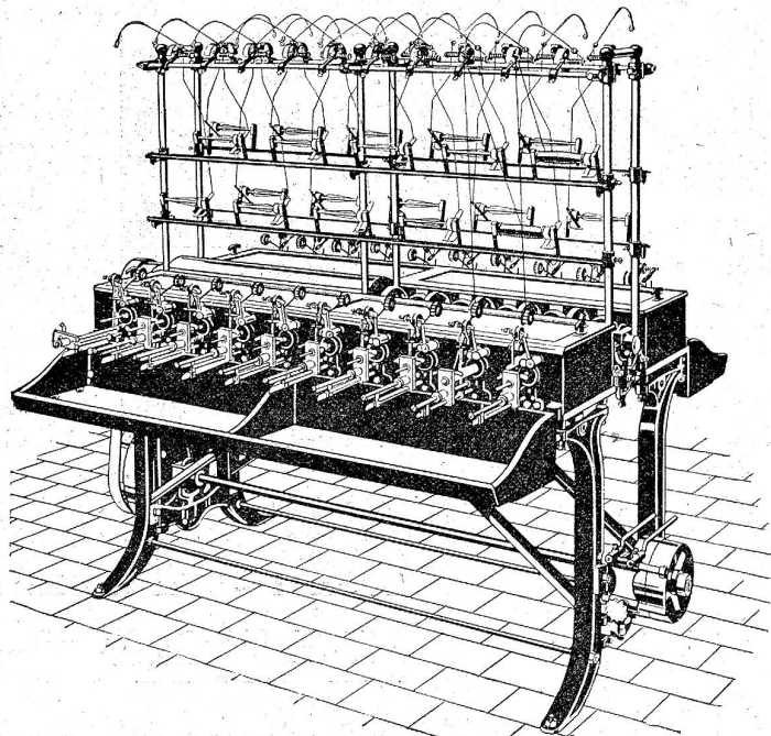
Kreuzschuß-Spulmaschine „Klein-Rapid“
