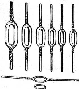
Universallitzen mit eingesetztem Stahrling
