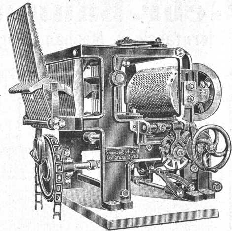
Doppelhub-Schaffmaschine „Reform“
