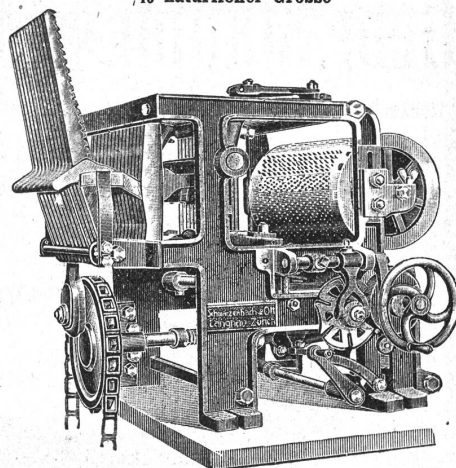
Doppelhub-Schaffmaschine „Reform“
