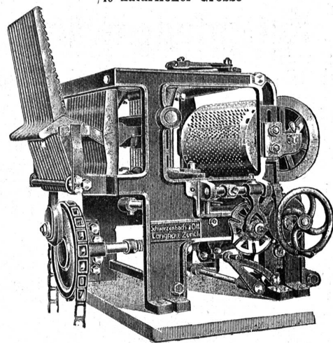
Doppelhub-Schaffmaschine „Reform“
