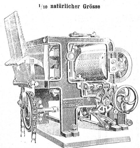
Doppelhub-Schaftmaschine „Reform“
