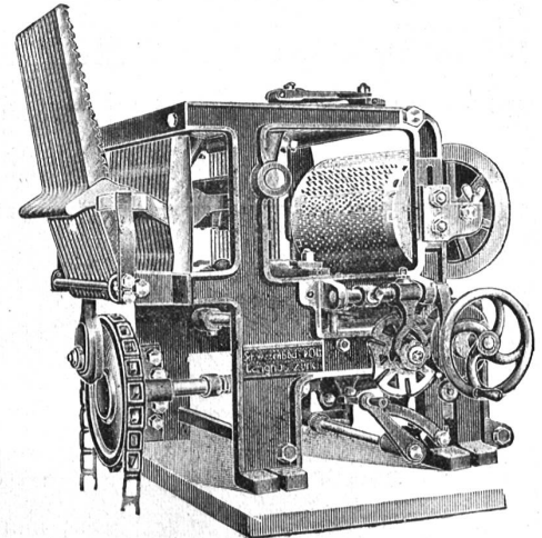
Doppelhub-Schaffmaschine „Reform“
