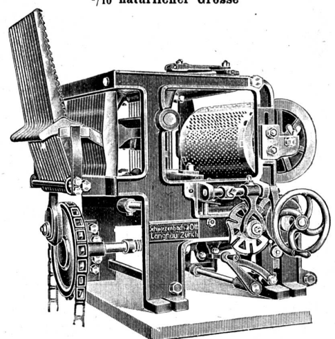
Doppelhub-Schaftmaschine „Reform“
