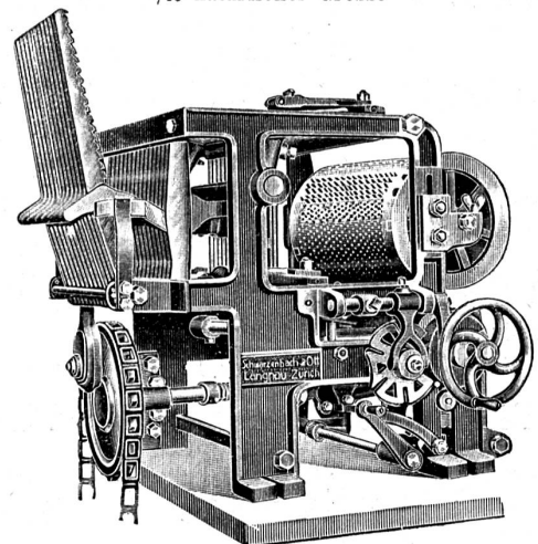
Doppelhub-Schaffmaschine „Reform“
