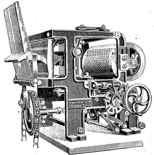
Doppelhub-Schaffmaschine „Reform“
