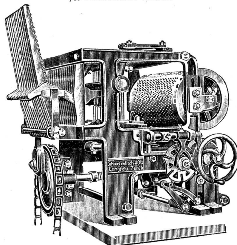
Doppelhub-Schaftmaschine „Reform“
