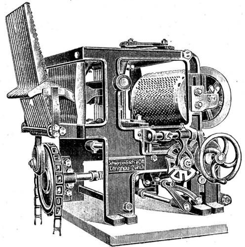
Doppelhub-Schaftmaschine „Reform“
