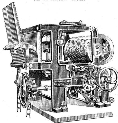
Doppelhub-Schaffmaschine „Reform“
