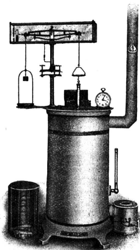
Gangbarste Grösse: Für Versuche bis 500 gr. und mehr. Zur Bestimmung des Feuchtigkeitsgehaltes loser Textil-Rohstoffe und Garne von Wolle, Seide, Baumwolle, (Papier-Rohstoffe, Holzschliff etc.). Für Spiritus-, Gas- oder elektrische Heizung. Neueste solide Ausführung mit feinsten Präzisions- Wage in metallgefasstem Glasgehäuse, Drahtkorb, Hakenkranz, Thermometer, Wasserwage, Gewichtssatz
