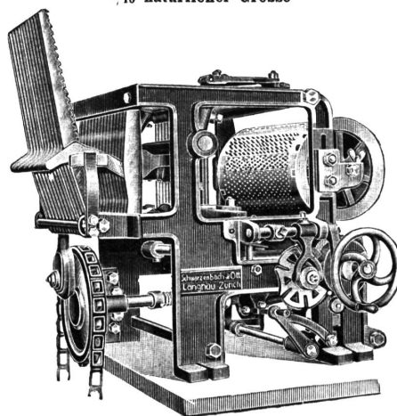
Doppelhub-Schaffmaschine „Reform“
