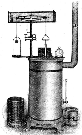
Gangharste Grösse: Für Versuche bis 500 gr. und mehr. Zur Bestimmung des Feuchtigkeitsgehaltes loser Textil-Rohstoffe und Garne von Wolle, Seide, Baumwolle, (Papier-Rohstoffe, Holzschliff etc.). Für Spiritus-, Gas- oder elektrische Heizung. Neueste solide Ausführung mit feinsten Präzisions- Wage in metallgefasstem Glasgehäuse, Drahtkorb, Hakenkranz, Thermometer, Wasserwage, Gewichtssatz
