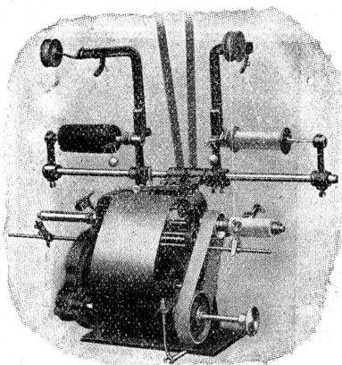
Präzisions-Kreuz-Spulmaschine à 2 Spindeln für Spulen bis 60 mm.
