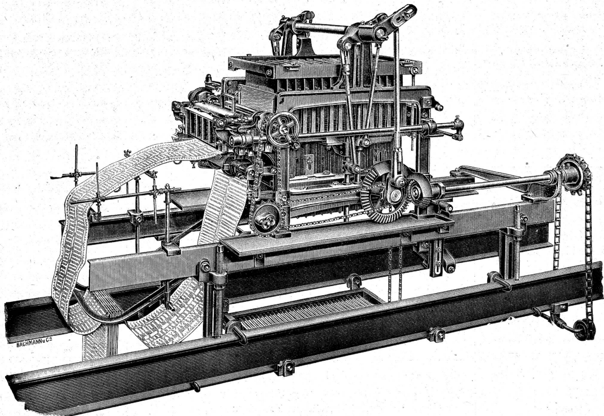
Doppelhub - Verdolmaschine
