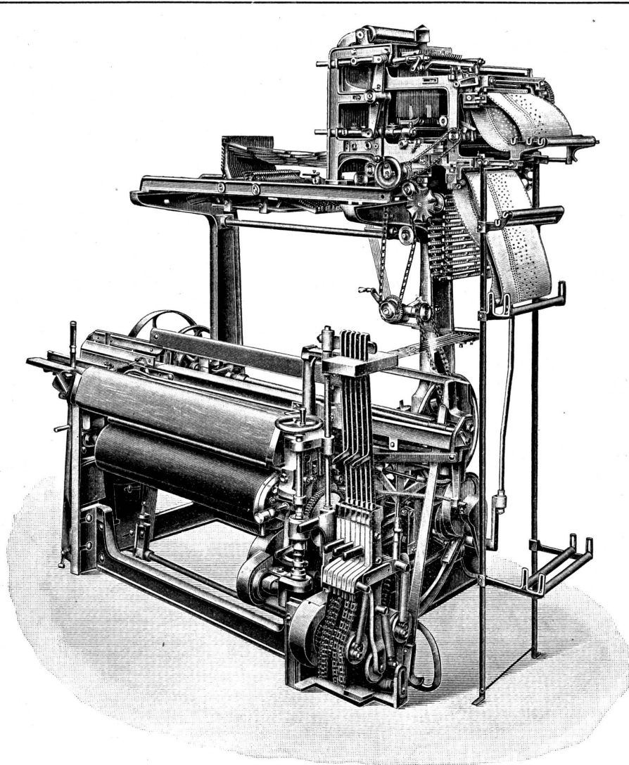
Seidenwebstuhl mit dreizylindriger Schaftmaschine und einseitig sechs- :: fachem Schützenwechsel ::
