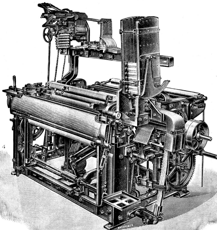
Mechanischer Webstuhl mit automatischem Schusspulwechsel
