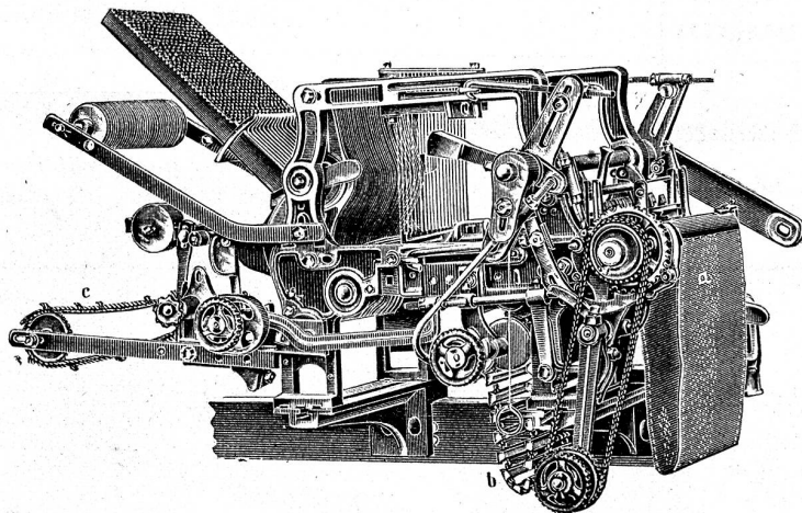
Zweckmässigste Maschine für sämtliche Droherstoffe und carrierte Gewebe mit Taffet- (Leinwand) Grund.
