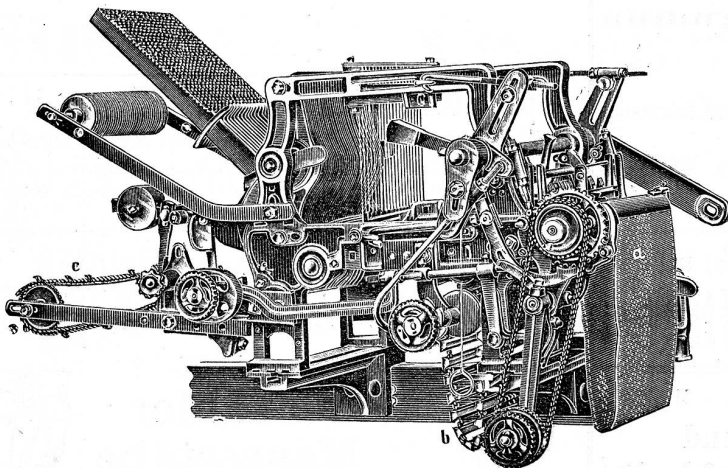
Zweckmässigste Maschine für sämtliche Dreherstoffe und carrierete Gewebe mit Taffet- (Leinwand) Grund.
