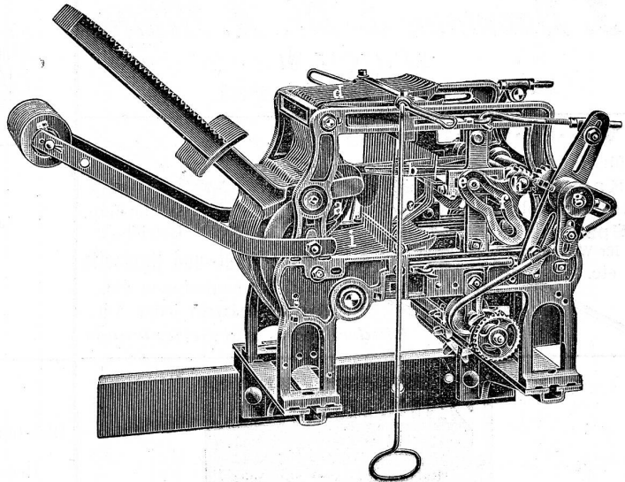
Zweckmässigste Maschine für sämtliche Dreherstoffe und carrierete Gewebe mit Taffet- (Leinwand) Grund.
