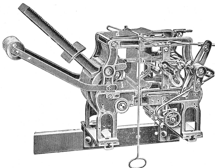
2 cylindrige Schaftmaschine
