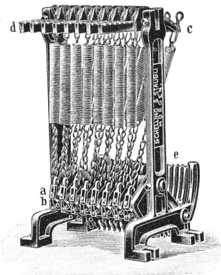
Federzugregister
