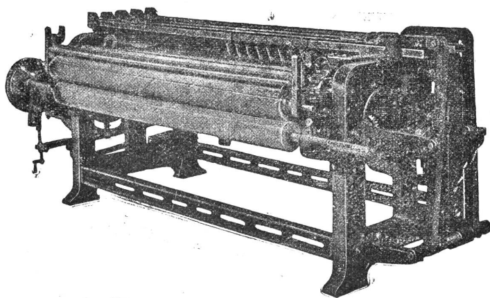
Reihmaschine gegen die Mitle reibend mit Messerschlitzen, System Simonin
