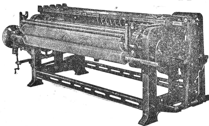
„Diese Reithmaschine gegen die Mille feilt mit Messerschiffen System Simonin“
