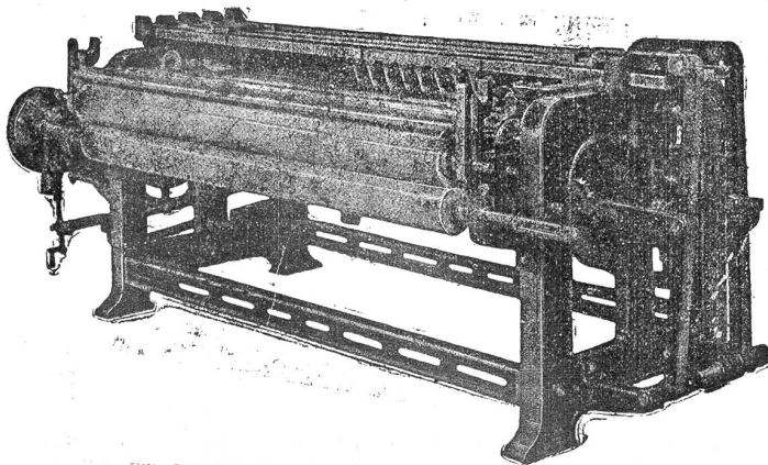
Neue Reibmaschine gegen die Mitternachtszeit Messerschmitt-System Simonin. Nouveaux machines à rebroussement avec chariot à l'usage des machines Simonin.
