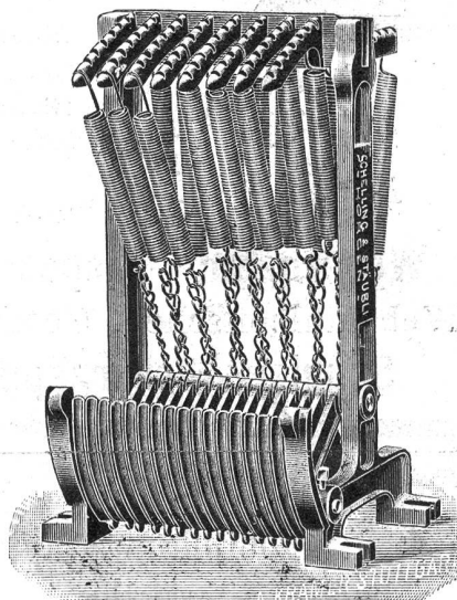
Federnzug-Register jeder einzelne Flügelzug beliebig regulirbar.
