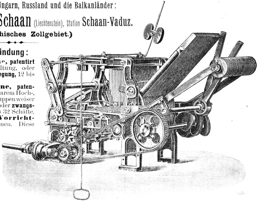
Offenfach Schaffmaschine, doppelhebend, mit zwangsläufiger Cylinderbewegung. Gros-de-tour-Vorrichtung und Hakenauskehrung.
