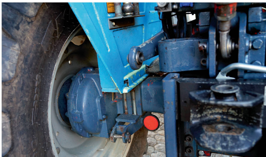
Grâce au pignon terminal, l'étrillage avec le « 6060 » s'effectue aisément sans lestage.
