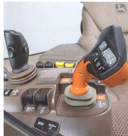
Le nouveau joystick «CommandPro» permet l'action intuitive sur de nombreuses commandes et fonctions du tracteur.
