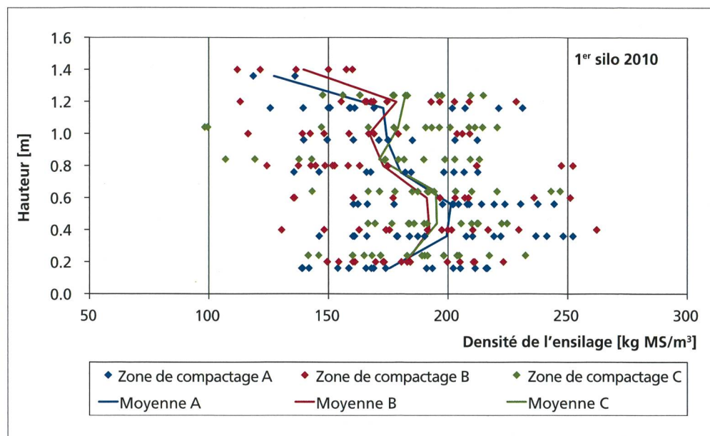
Fig. 2: Répartition des valeurs de densité dans le 1 er silo en fonction de la hauteur des prélèvements.
