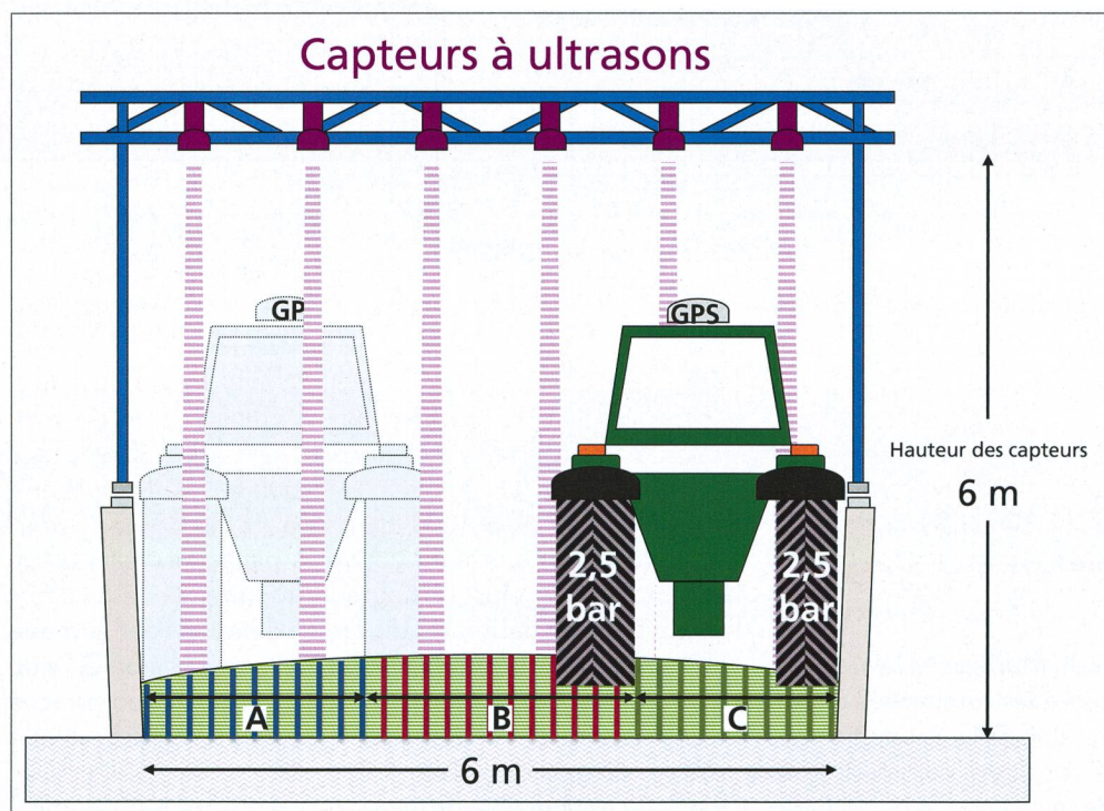
Fig. 1 : Schéma de l'essai avec capteurs à ultrasons, pneus de différentes largeurs et zones de compactage A, B et C en fonction des pneus. Dans la zone B, les temps de compactage des zones A et C s'additionnent, il est donc deux fois plus élevé.
