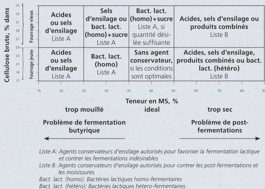
Fig. 3: Schéma du choix d'un agent conservateur pour l'herbe (modifié selon Nussbaum)
