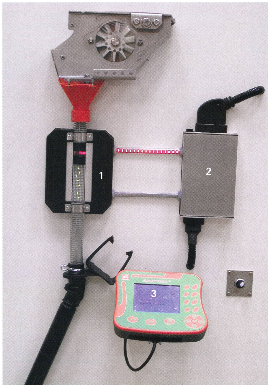
Fig. 5: Le capteur optique (1) intégré dans la conduite de semis, avec ordinateur de bord (2) et terminal ISO-Bus (3) permet l'arrêt automatique de la machine et la régulation spécifique de la densité de semis.
