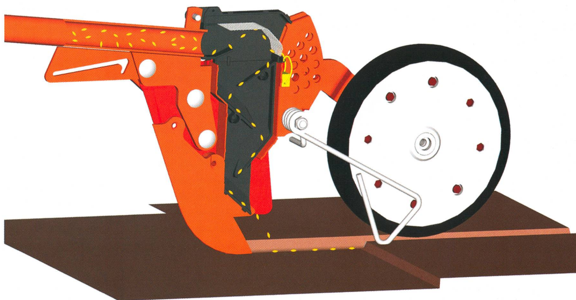
Fig. 3: Le soc en cascade de Kuhn, à l'origine un développement de l'Uni de Hohenheim, améliore la répartition dans le sillon, ce qui amène une réduction du volume de semences de 10-15%.
