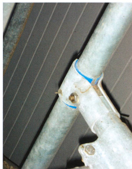
La pose de manchons en plastique aux points de croisement des conduites garantit un effet isolateur.
