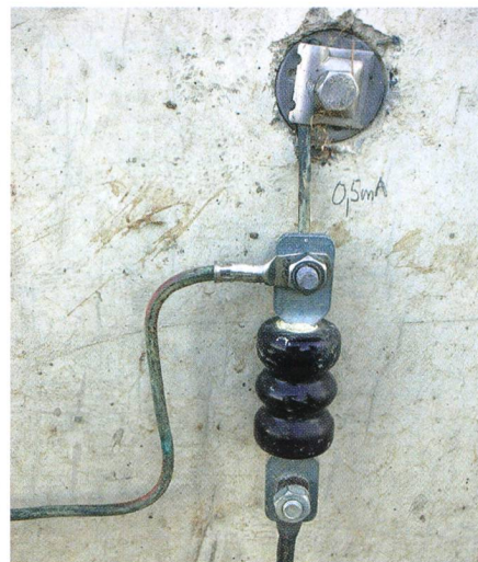
L'éclateur de paratonnerre joue un rôle tampon entre le paratonnerre et les autres structures métalliques.
