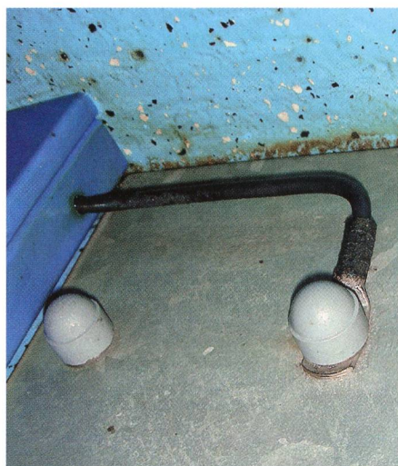
En reliant les parties métalliques à la mise à terre, on dévie les courants vagabonds en direction du sous-sol.
