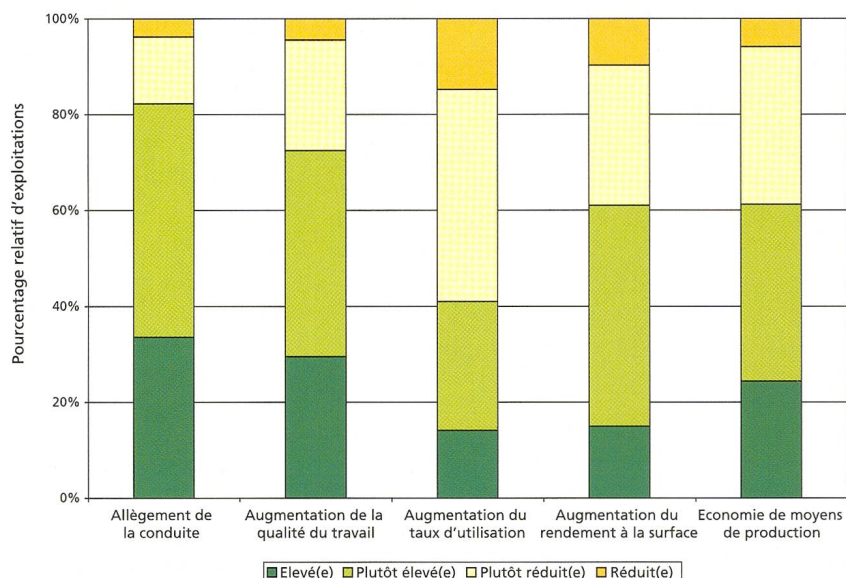
Fig. 3: Influence des composants électroniques supplémentaires du tracteur, sur l'allègement de la conduite, l'augmentation de la qualité du travail, du taux d'utilisation, du rendement à la surface et sur l'économie de moyens de production.
