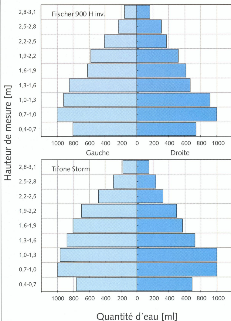
Fig. 5: En haut: Deux bancs d'essais à lamelles FAT permettent d'optimiser le réglage de base du pulvérisateur par rapport à la forme de l'arbre. A gauche: Exemples de répartition verticale d'eau. A droite: bien qu'on ait prévu une quantité plus faible d'eau dans la zone supérieure, pratiquement toutes les niveaux de mesure dans l'arbre affichent soit une bonne couverture foliaire, soit une couverture hétérogène (avec/sans déflecteur).
