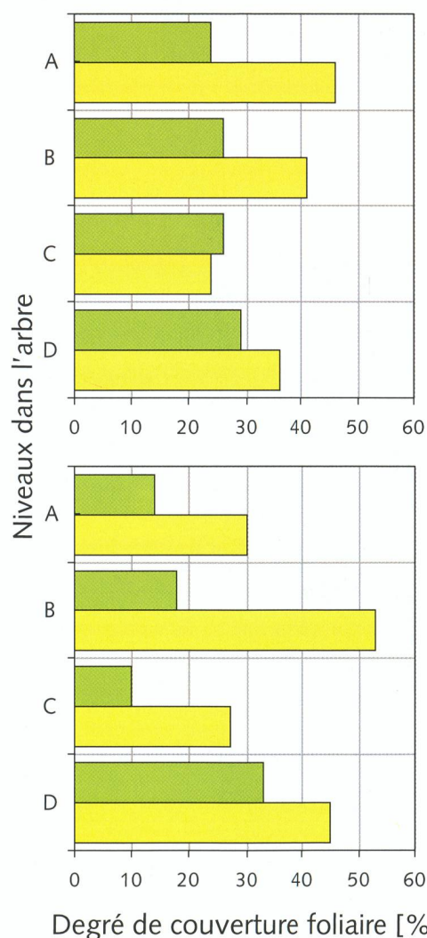
Fig. 5: En haut: Deux bancs d'essais à lamelles FAT permettent d'optimiser le réglage de base du pulvérisateur par rapport à la forme de l'arbre. A gauche: Exemples de répartition verticale d'eau. A droite: bien qu'on ait prévu une quantité plus faible d'eau dans la zone supérieure, pratiquement toutes les niveaux de mesure dans l'arbre affichent soit une bonne couverture foliaire, soit une couverture hétérogène (avec/sans déflecteur).
