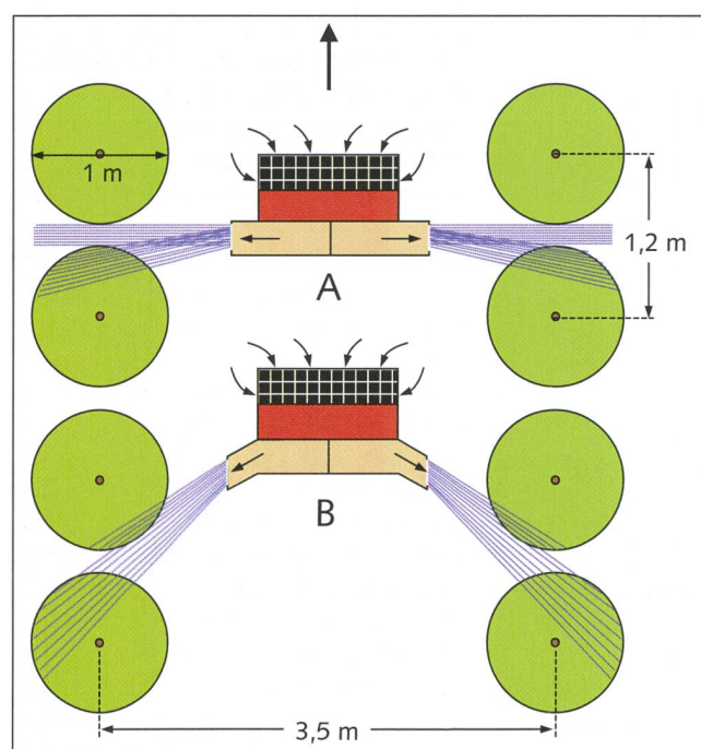
Fig. 10: Schéma du mode de fonctionnement du pulvérisateur avec souffleuse axiale inversée:
