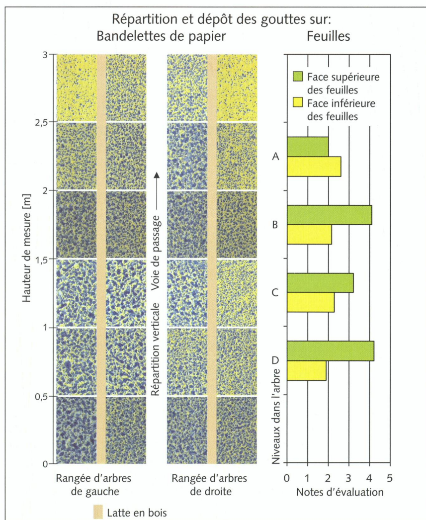
Fig. 8: Répartition verticale et dépôt des gouttes sur les feuilles (Fischer).
