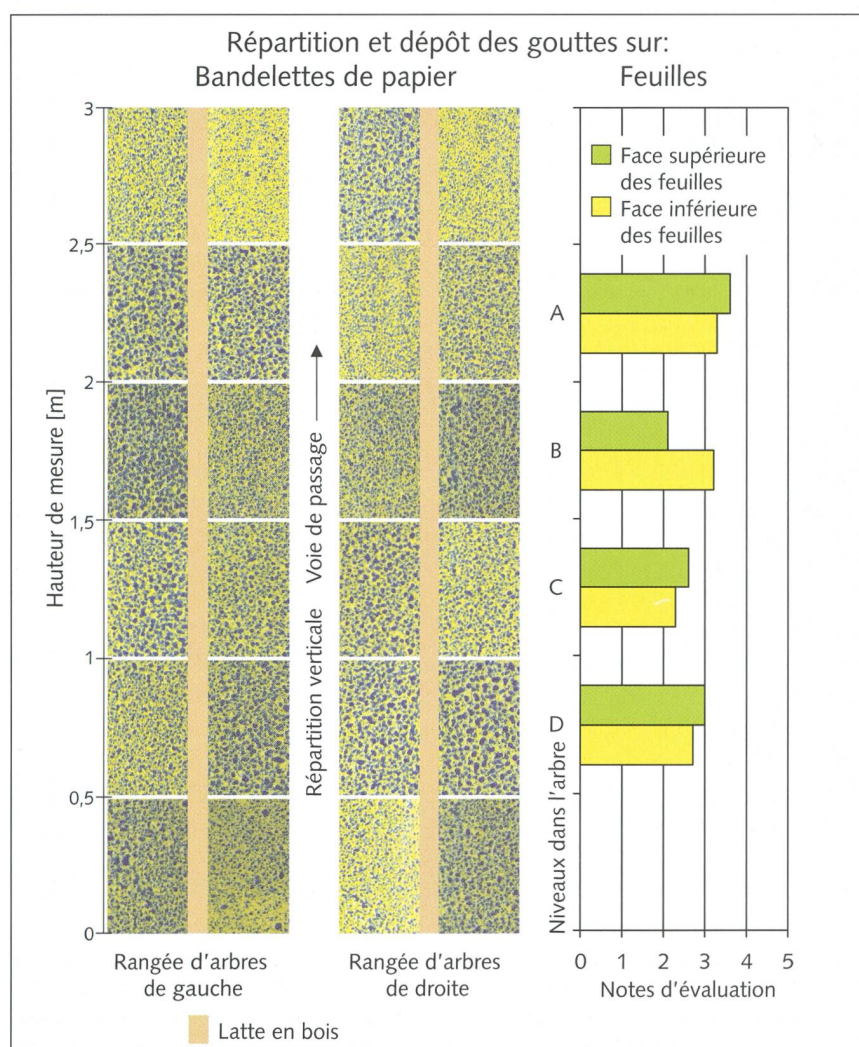
Fig. 7: a) Répartition verticale et dépôt des gouttes sur les feuilles (Tifone).
