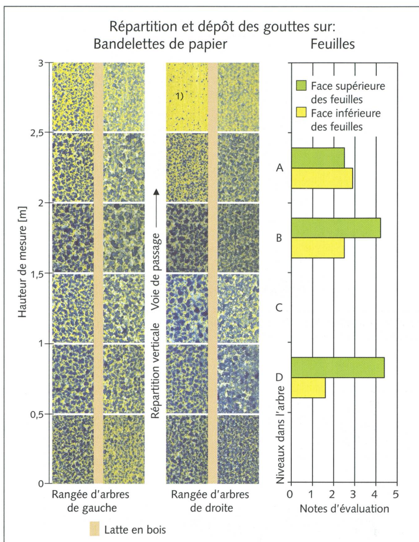
Fig. 9: Répartition verticale et dépôt des gouttes sur les feuilles (Berthoud).
