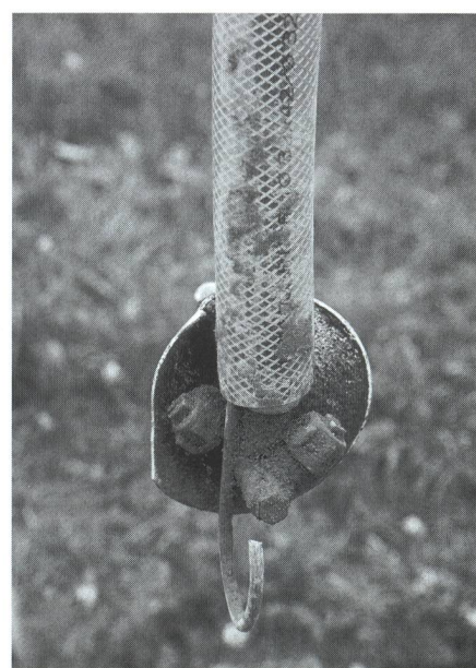
Fig. 6: Les supports de buses, suspendus sur ressorts sont réglables horizontalement et verticalement sur la perche du pulvérisateur (Fischer, prototype 2). A droite: le dispositif de protection de la buse, en forme de cône, s'est avéré satisfaisant, mais doit encore être amélioré.
