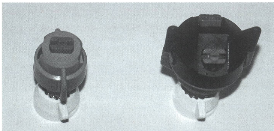
Fig. 3: Les buses à injection d'air, à jet plat, individuelles et doubles se caractérisent par des gouttes relativement grossières, peu sujettes à la dérive et par une importante plage de pression (Agrotop de U. Wyss, Bützberg).
