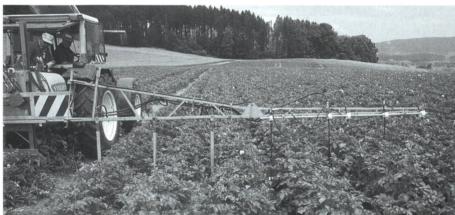
Fig. 1: Des pulvérisations ciblées, appliquées à temps depuis les voies de passage suffisent généralement à protéger les pommes de terre du mildiou. En bas: les meilleurs résultats ont été obtenus avec le dispositif de pulvérisation sous-foliaire (prototype).
