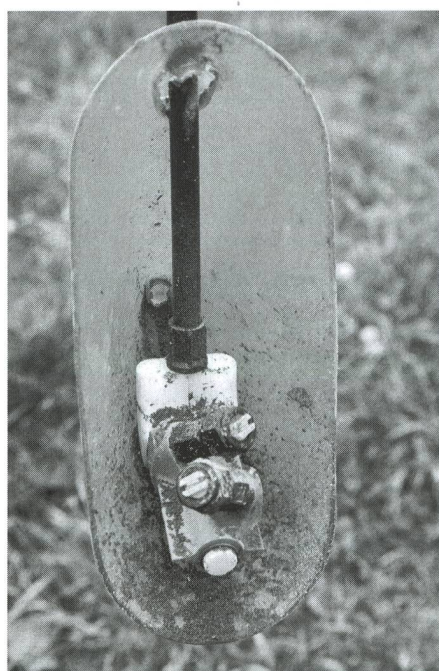
Fig. 7: Les supports de conduits en plastique relativement souples peuvent être réglés et fixés (Birchmeier, prototype 1). En bas: les buses doubles bien placées nécessitent une protection compacte et des supports plus stables.
