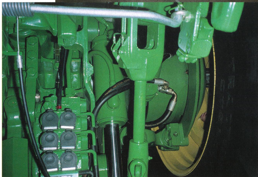
Prototype de la nouvelle suspension arrière pour la future série 8020.
