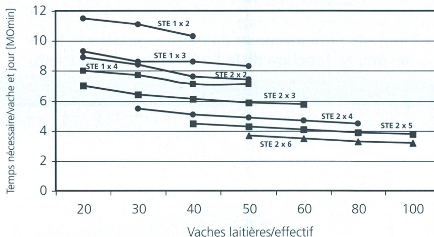
Fig. 9: Dans les salles de traite en épi, suivant l'équipement disponible, il est possible d'économiser plus de huit minutes par vache et par jour.
