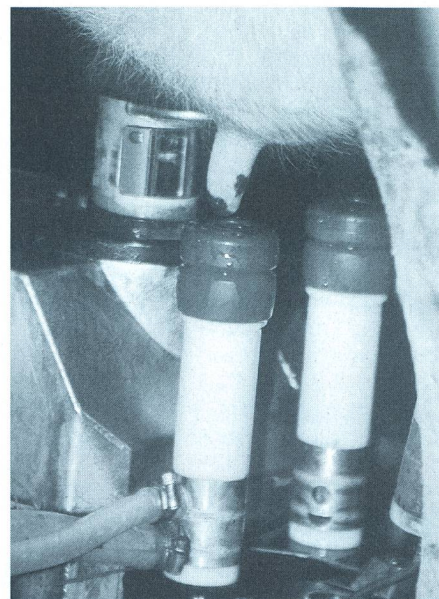
Fig. 17: Dans les systèmes de traite automatiques, tous les travaux routiniers sont effectués automatiquement lorsque le dispositif fonctionne parfaitement. Par contre, les opérations de contrôle sont considérables.
