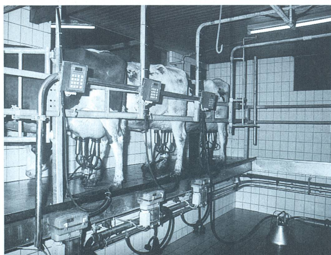
Fig. 14: La salle de traite en épi réunit plusieurs avantages: faible place occupée, déplacements relativement courts et bonne vue d'ensemble du pis des vaches.
