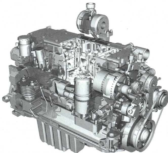
Fig. 1: Moteur diesel moderne DEUTZ, type BF6M 2013, 6 cylindres, cylindrée 5,7 litres, 4 soupapes par cylindre. L'injection se réalise par une pompe d'injection individuelle, une conduite et des buses. Le système de turbocompression est équipé d'un refroidissement d'air de suralimentation placé en aval. Ce moteur se caractérise par une souplesse élevée, une consommation faible et des émissions de bruit et de gaz d'échappement favorables. Il équipe le FENDT Favorit 716 Vario, Test FAT no 1792/99.
