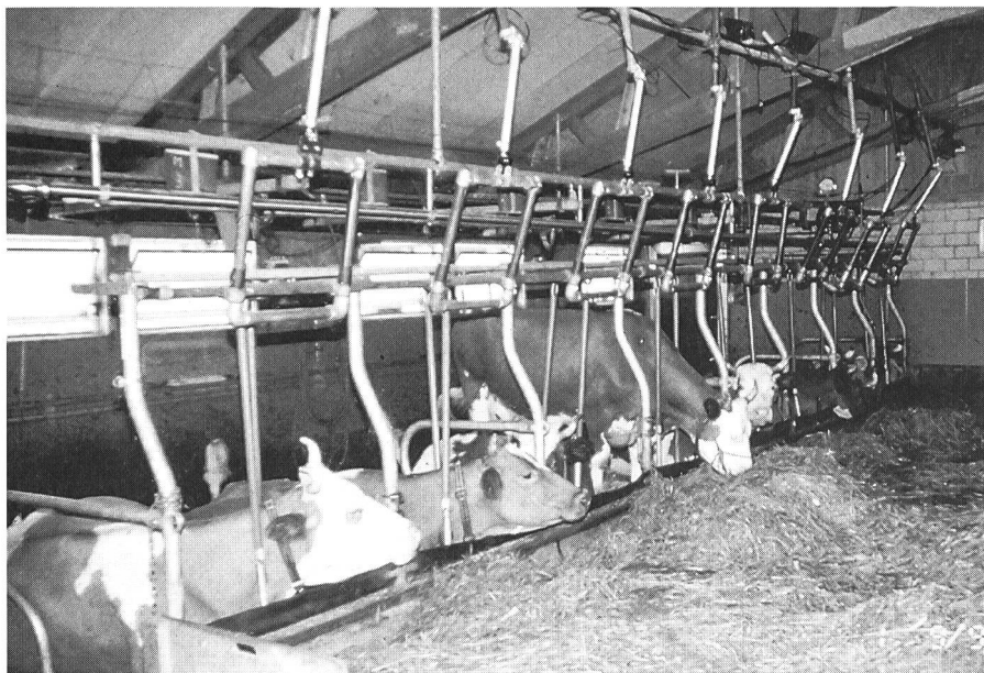
Photos 7, 8. L'arceau à commande pneumatique à mouvement rectiligne et point d'impact sur la nuque s'est avéré très efficace.
