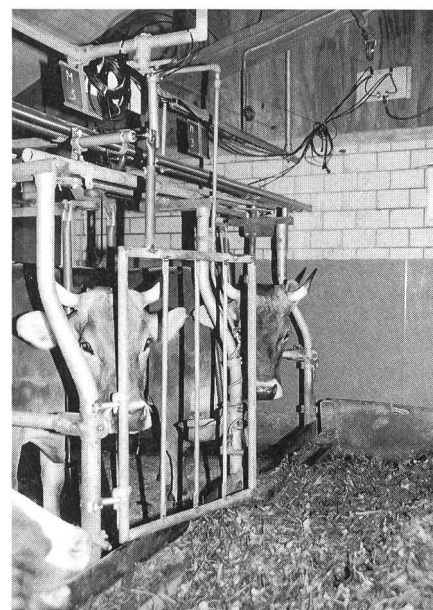
Photo 3. Lorsque la vache défèque ou urine, la crèche est fermée pneumatiquement. L'efficacité de ce système s'est avérée satisfaisante.
