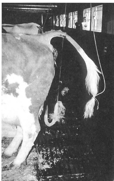
Photos 13, 14, 15. Lorsqu'elle défèque ou urine, la vache lève la queue et supprime la pression qui s'exerce sur l'attache-queue. Ce signal est enregistré par un capteur et transmis à un dispositif électronique d'évaluation. Celui-ci transmet ensuite le signal au mécanisme.
