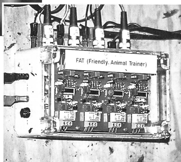
Photos 13, 14, 15. Lorsqu'elle défèque ou urine, la vache lève la queue et supprime la pression qui s'exerce sur l'attache-queue. Ce signal est enregistré par un capteur et transmis à un dispositif électronique d'évaluation. Celui-ci transmet ensuite le signal au mécanisme.
