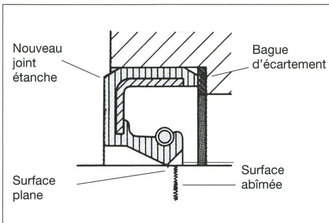
Réparation sans douilles de protection: En premier lieu s'assurer qu'il y aura suffisamment d'espace sur les côtés. Ensuite placer le nouveau joint avec une bague d'écartement. (Croquis publiés avec l'autorisation de la maison SKF.)
