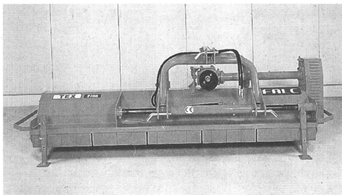
TEX avec réglage latérale hydraulique.
