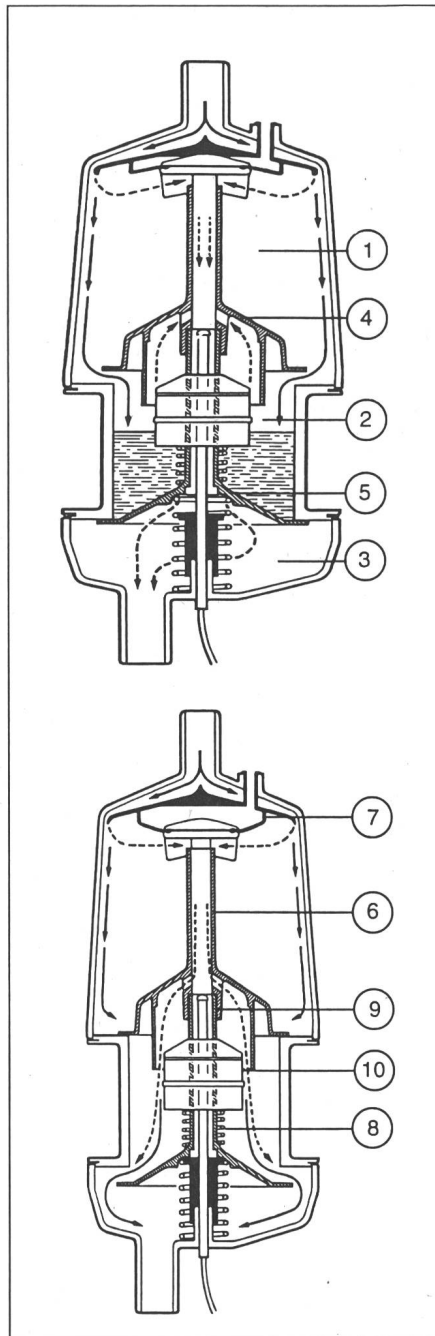
Fig. 15. Coupe des principaux éléments fonctionnels du Manuflow 2:
