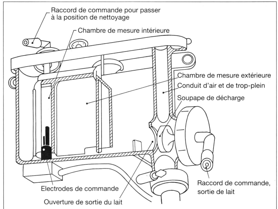
Fig. 13. Coupe des éléments fonctionnels du Metatron 12.
