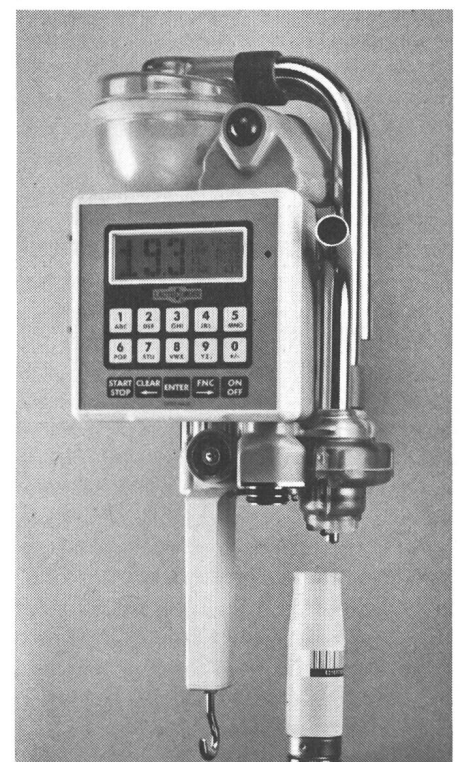
Fig. 5. LactoCorder: l'appareil est actuellement testé auprès du CICPE; la décision est en suspens.
