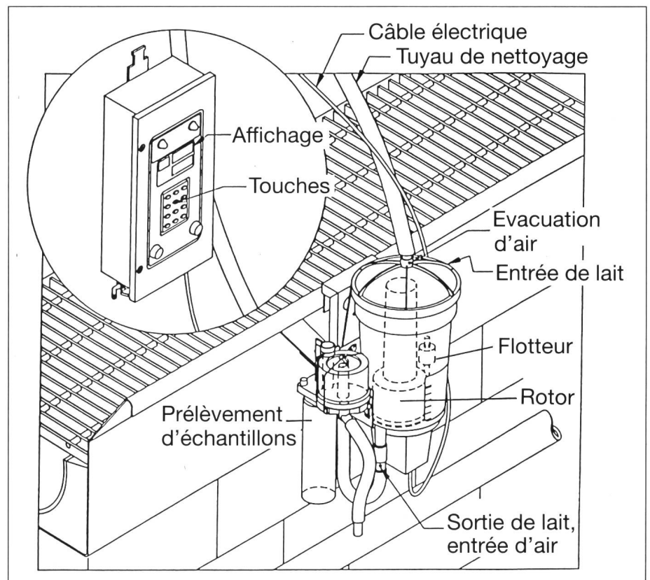
Fig. 14. Bou-Matic M+ avec dispositif de prélèvement d'échantillons.
