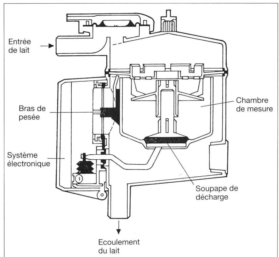
Fig. 9. Représentation schématique du Flo Master 2000.
