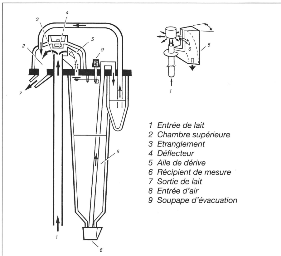
Fig. 4. Les principaux éléments fonctionnels du Milkoscope MK II:
