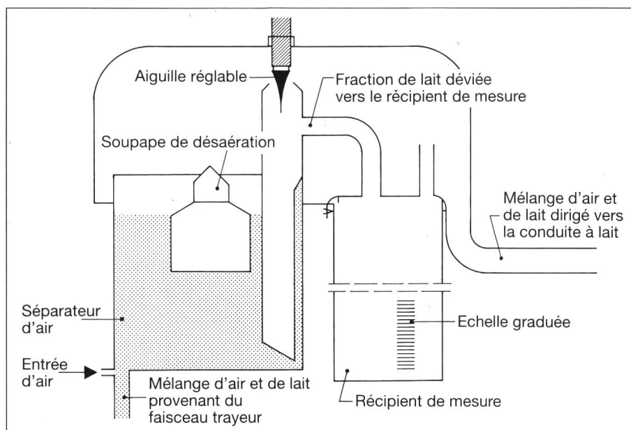
Fig. 6. Eléments fonctionnels du Milkoskope I.
