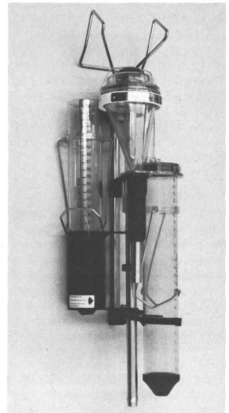
Fig. 3. Tru-Test HI (avec cylindre de mesure interchangeable): autorisé pour les installations de traite en lactoduc dans les étables à stabulation entravée aussi bien qu'en salle de traite.
