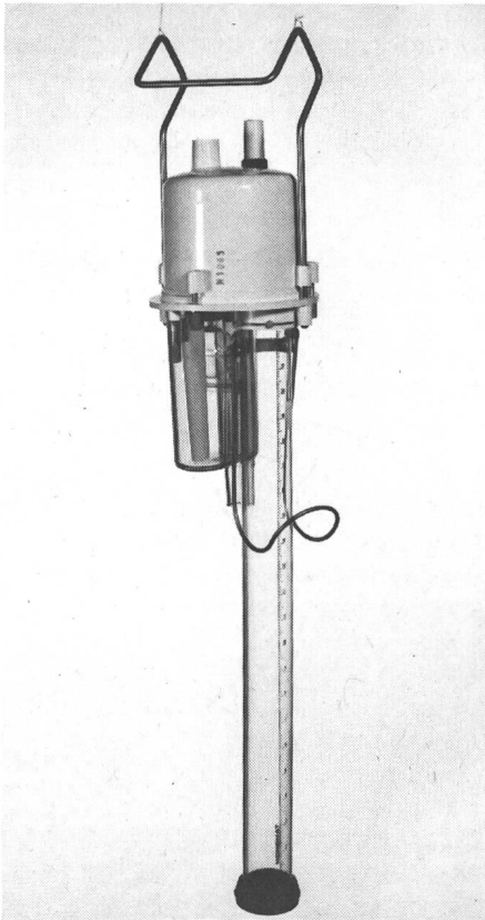
Fig. 1. Milkoscope I: seuls les appareils déjà en service sont autorisés; de nouvelles acquisitions ne sont pas admises.
