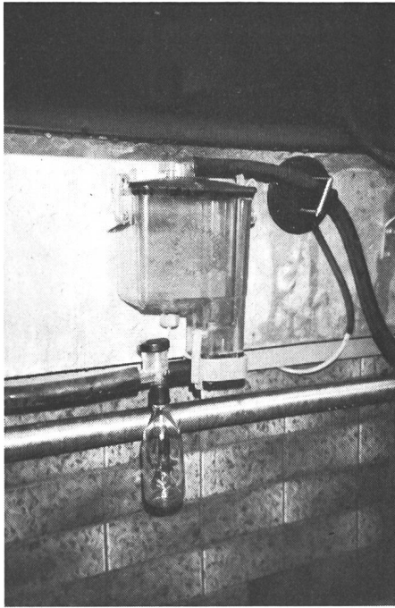
Fig. 10. Le Fullflow Milkmeter (identique au Nyflow 85) avec flacon d'analyse.
