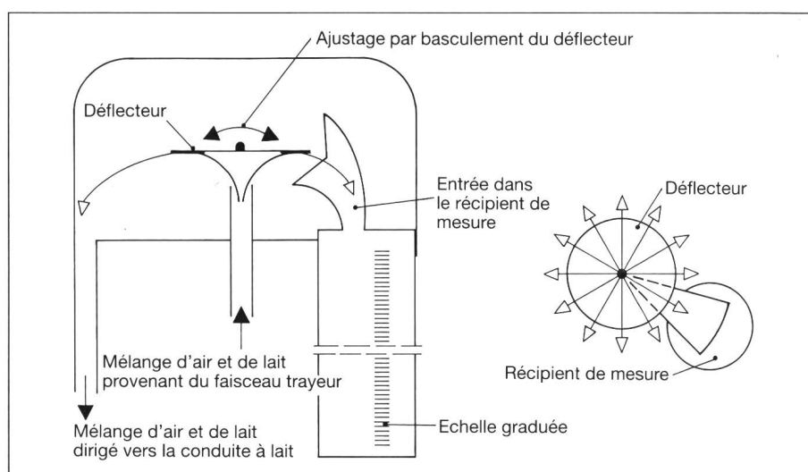
Fig. 7. Représentation schématique des compteurs à lait travaillant en continu et pourvus d'un déflecteur pour collecter une fraction du lait traité. Le Milkoskope II, le Tru-Test HI et le Milkoskope MK II appartiennent à cette catégorie d'appareils.
