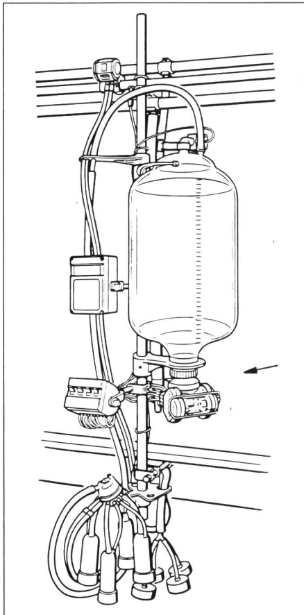
Fig. 12. Le JM 100 est fixé au fond du récipient de mesure (flèche). Le lait de chaque vache est collecté dans le récipient de mesure; il n'est évacué par la pompe qu'après que le faisceau trayeur a été décroché. L'appareil fonctionne selon le principe d'une pompe à piston avec un volume défini de 100 ml par course.
