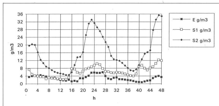
Fig. 5. Déroulement de l'essai No 5. La quantité spécifique d'eau extraite (E) évolue, au cours des 48 heures de la durée de séchage, parallèlement au déficit de saturation (S2) mesuré après la pompe à chaleur. La «capacité de travail» de la pompe à chaleur dépend des conditions météorologiques, c'est-à-dire du déficit de saturation (S1) de l'air ambiant.
