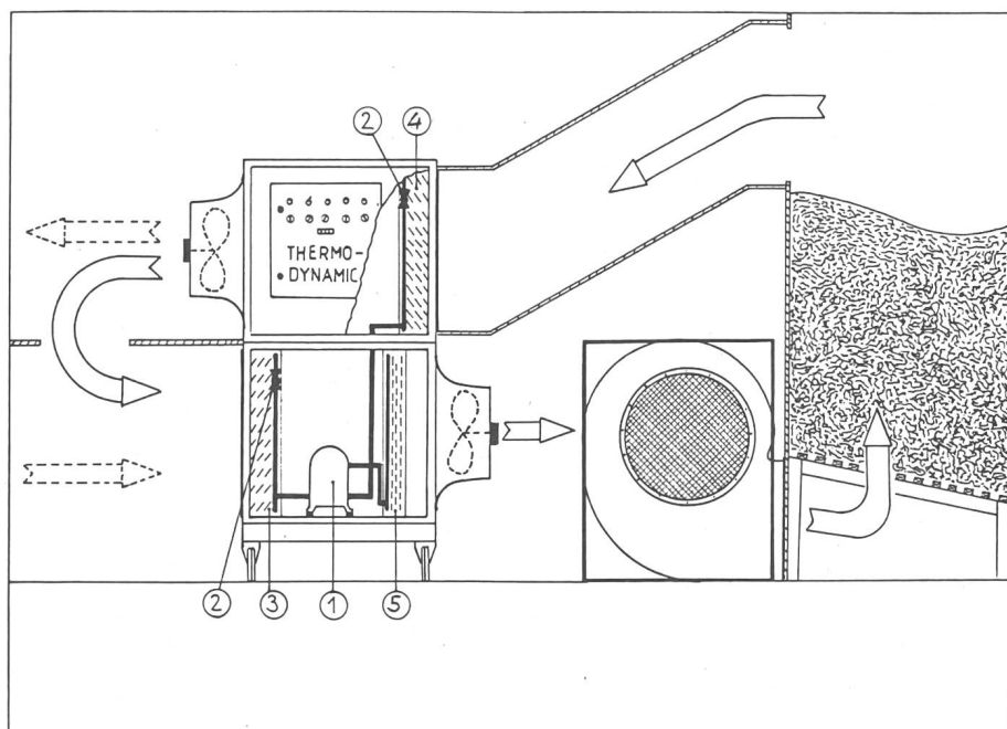
Fig. 2. Schéma de la pompe à chaleur: 1 = compresseur avec cuve sous pression, 2 = bobine, 3 = élément de refroidissement inférieur pour la déshumidification de l'air, 4 = élément de refroidissement supérieur pour la récupération de la chaleur contenue dans l'air qui se dégage du tas, 5 = radiateur de chauffage.
