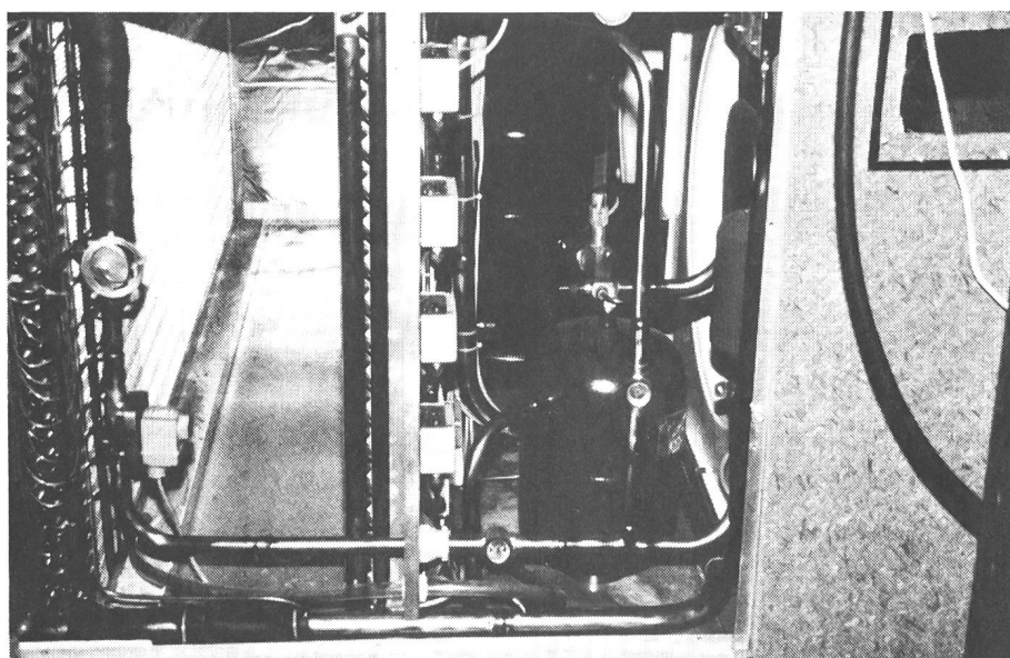
Fig. 1. Vue de l'intérieur de la pompe à chaleur. Les principaux éléments sont, de gauche à droite: l'élément de refroidissement, le radiateur de chauffage et le compresseur avec la cuve sous pression.
