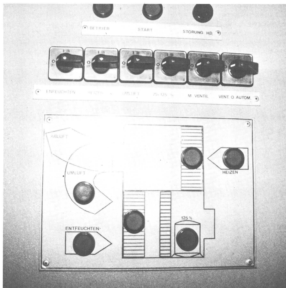
Fig. 3. Il existe différents modes de fonctionnement. Ils sont représentés par des symboles et des ampoules-témoin. Les témoins lumineux de fonctionnement et de dérangements facilitent le travail de l'exploitant.
