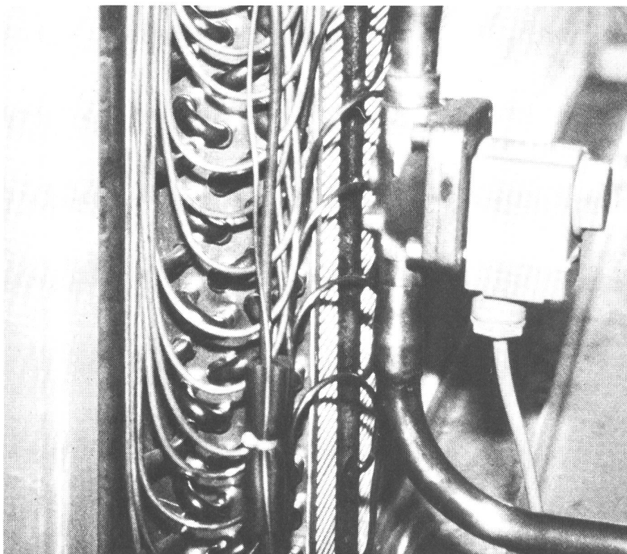
Fig. 4. L'échange de chaleur nécessite une technique coûteuse. L'encrassement des lamelles diminue le transport de chaleur et augmente la résistance que les éléments opposent à la circulation de l'air.
